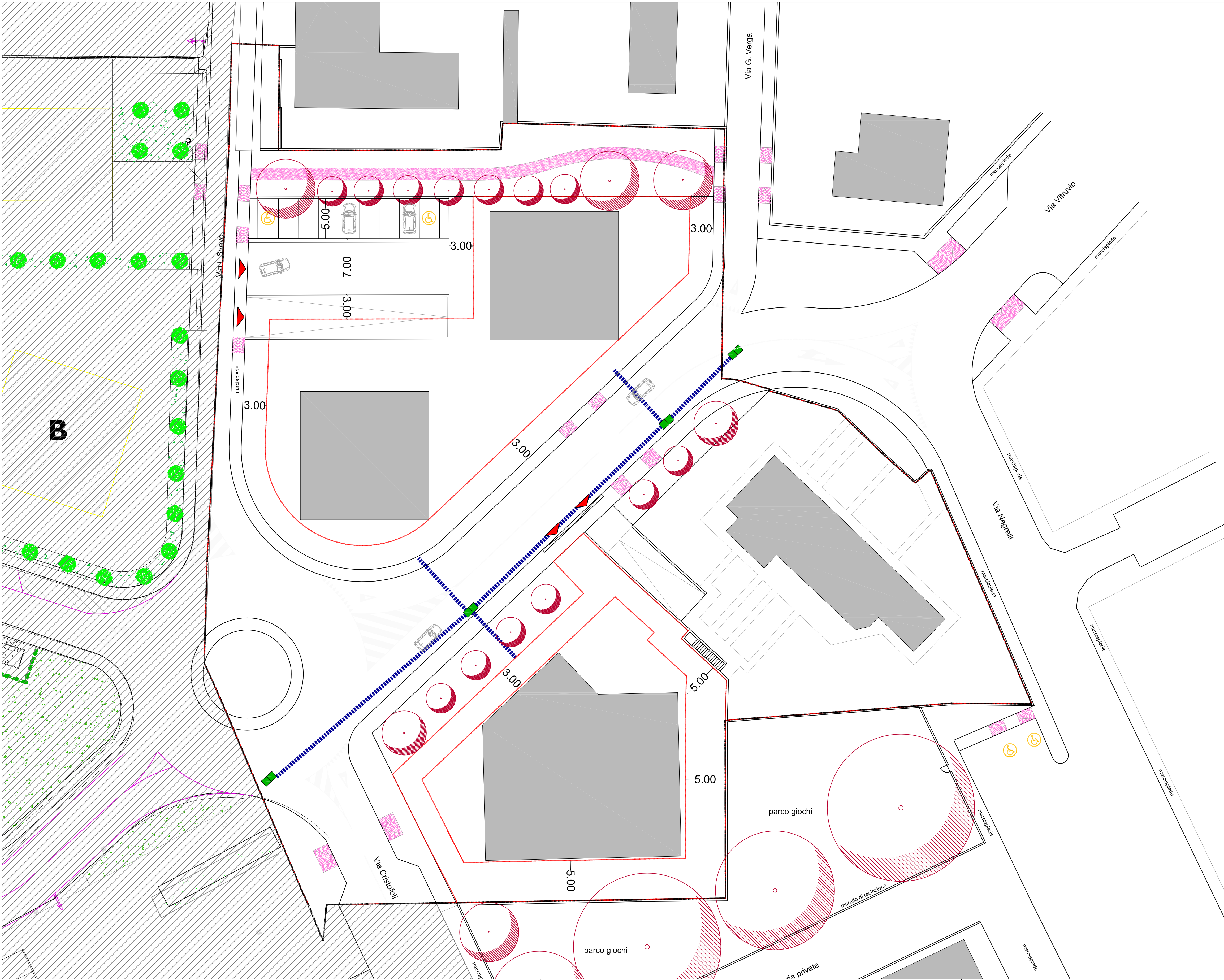
PLANIMETRIA AREA DI PROGETTO Scala 1:250
